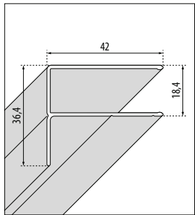
WALL G+FL - 3P - S - B - G
