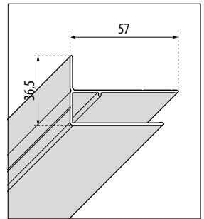
EXTENSION G+FL - 3P - S - B - G
